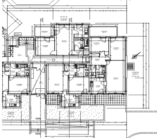
Plan d'exécution
