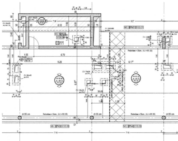
Plan d'exécution
